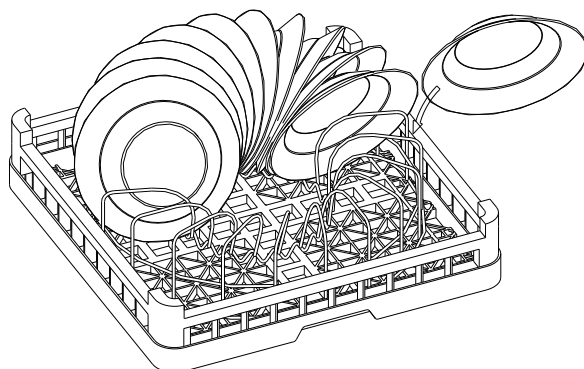
Rys.6e - Kosz do talerzy płatkich - 20 talerzy w koszu ( podstawa PB100 z wkładem PA200 )
