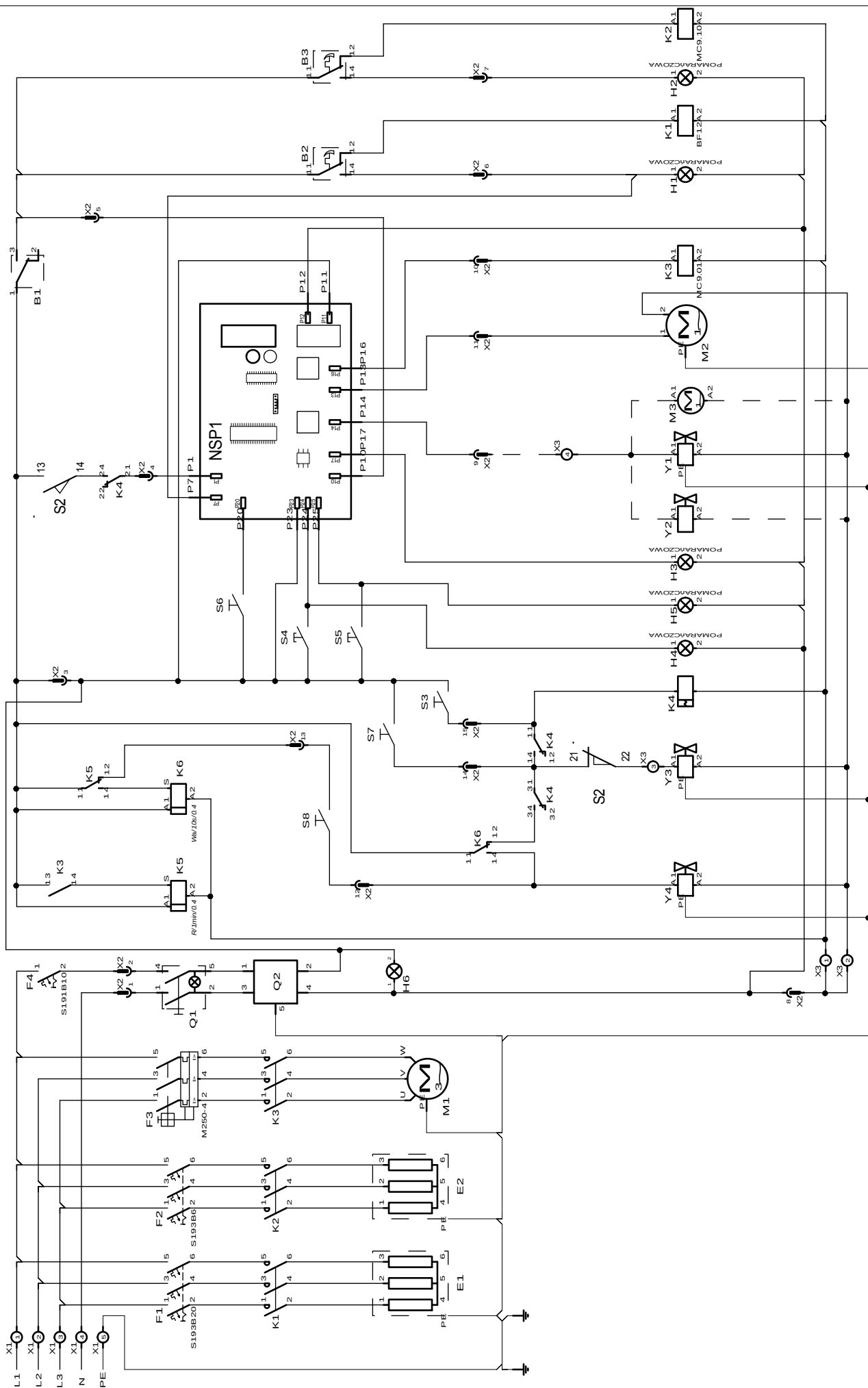
Rysunek 15 - Schemat elektryczny zmywarki ZKU-10.20EP
