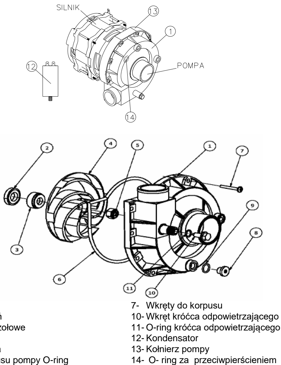
Rys. 19a - Pompa kompletna
