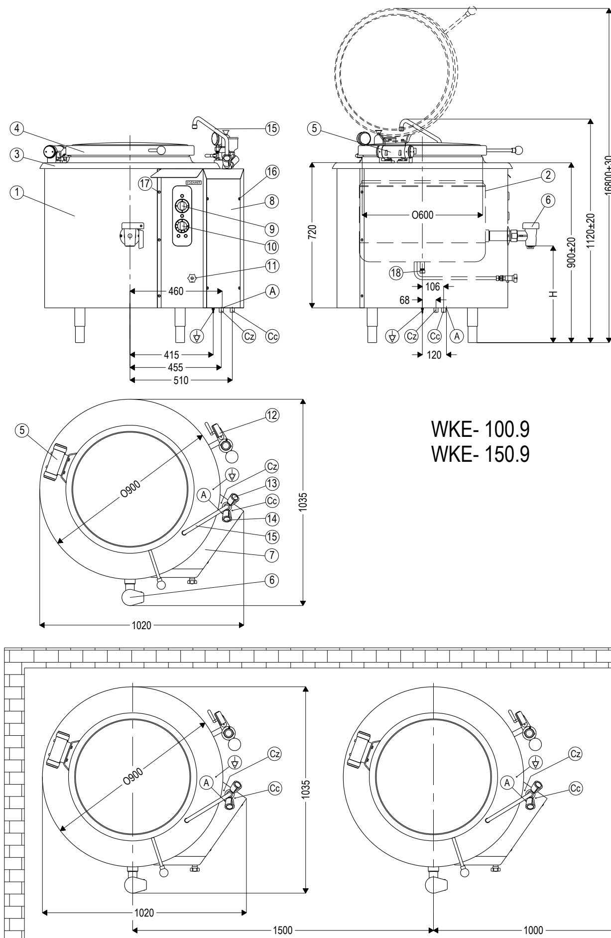
Rysunek 1 - Ogólny widok kotła
